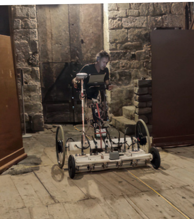
Prospecció amb georadar a l'interior de l'església de Sant Feliu de Barruera // PROCEDÈNCIA: Servei de Patrimoni Arquitectònic.
