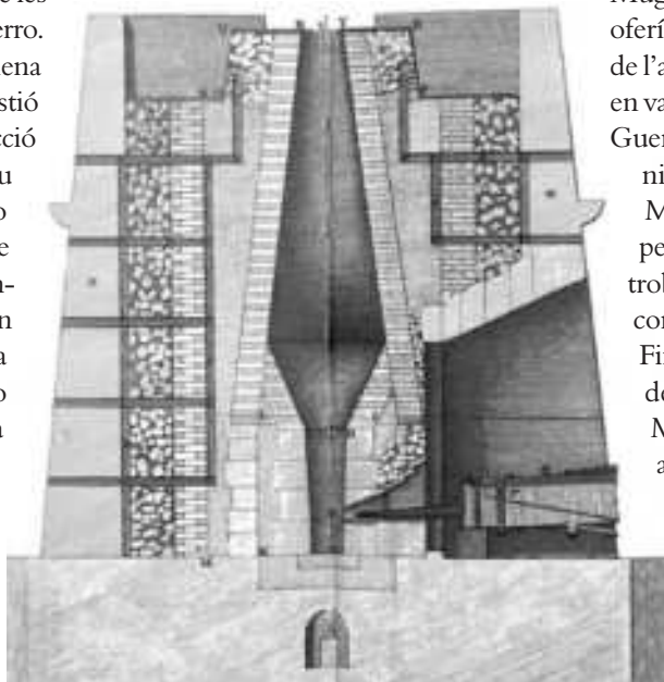
Secció de l'alt forn de la reial foneria de Sant Sebastià de la Muga, publicada en el 'Tratado de Artillería' de Tomás de Morla (1784).
